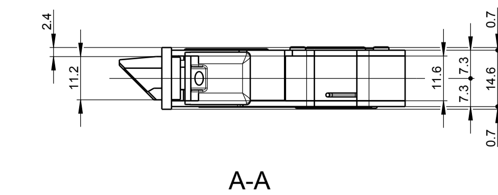
A-A
