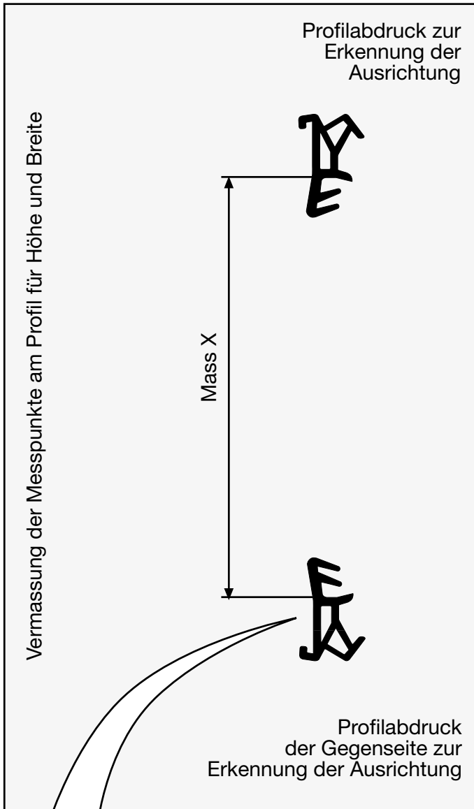
Beispiel 1 Flügeldichtung
