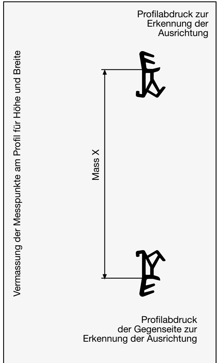
Beispiel 2 Rahmendichtung
