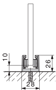
Variantes de guides inférieurs
