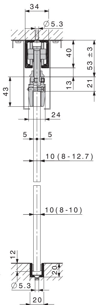
HAWA-Junior 80/GS
