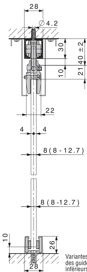
HAWA-Junior 40/GS
