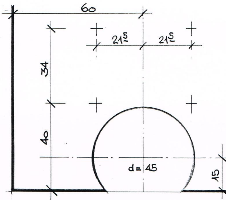
ANSICHT FRONT
