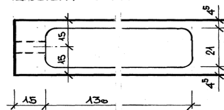
ANSICHT LINTEN
