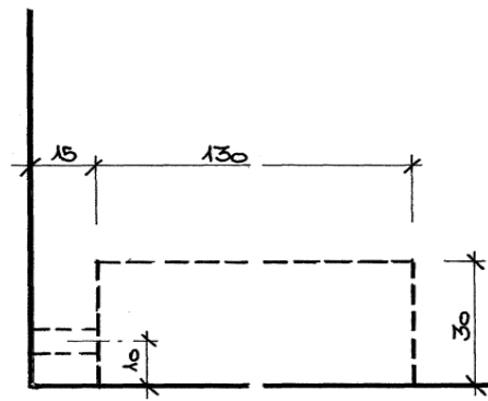
ANSICHT FRONT
