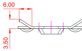
Ansicht E - F
