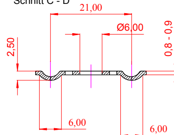
Schnitt C - D
