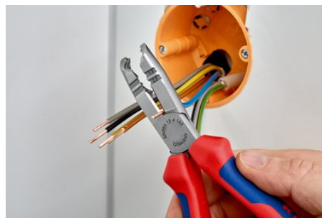
taglia quando si accorciano conduttori singoli
