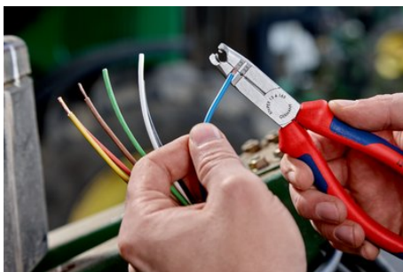
Fori di spelatura per conduttori da 1,5 e 2,5 mm 2
