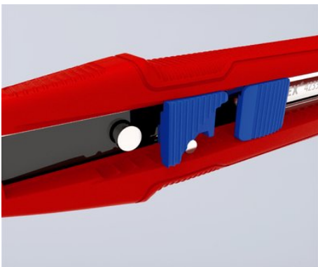
Zugstabile Klingerverriegelung und Klingensicherungsstift aus gehärtetem Stahl
