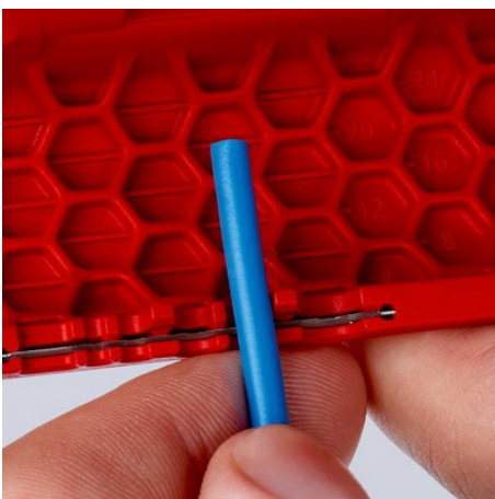
90 22 02 SB: Scala di lunghezza stampata a iniezione per una spelatura uniforme alla stessa lunghezza, leggibile per destrimano e mancini
