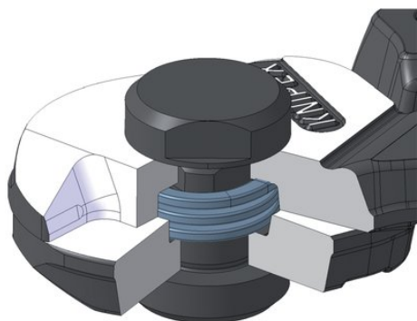
molla di apertura inserita nell'articolazione
