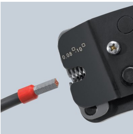
197 53 08 und 09: Vierkant-Crimp mit automatischer Größenanpassung!
