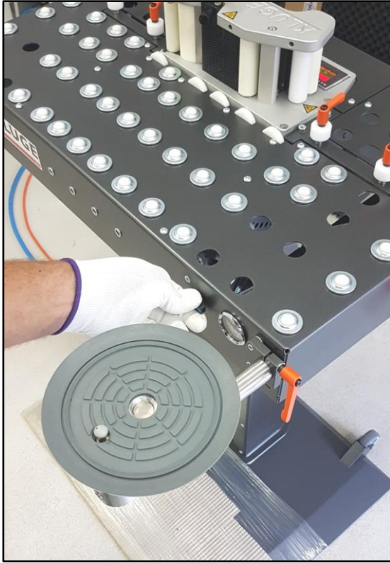
Abbildung 18 - Vakuumventil
