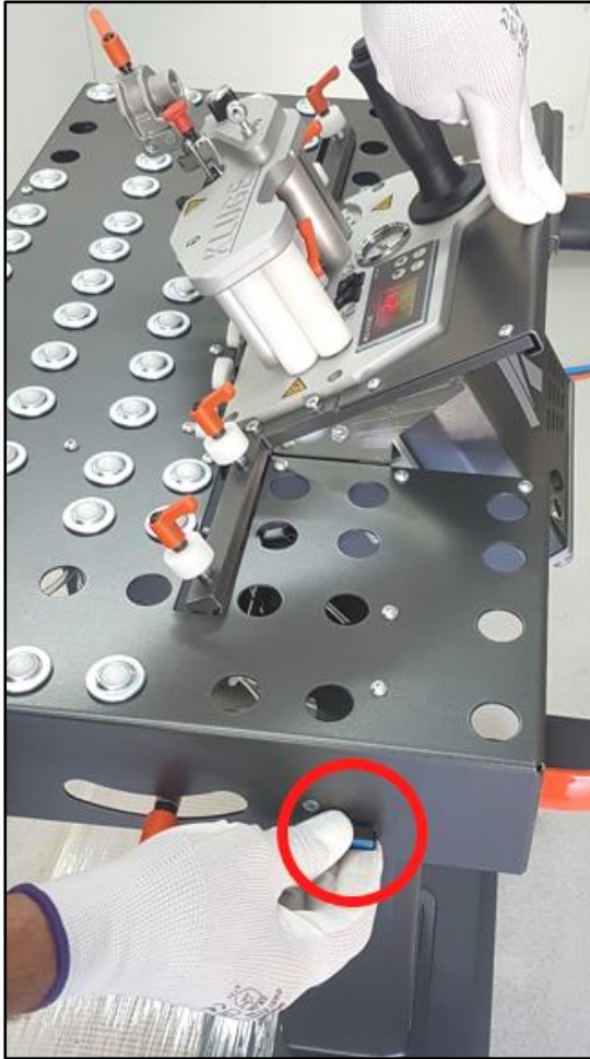
Abbildung 16 - Winkelverstellung
