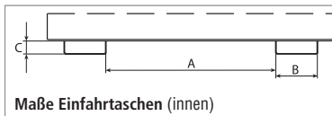
Maße Einfahrtaschen (innen)
