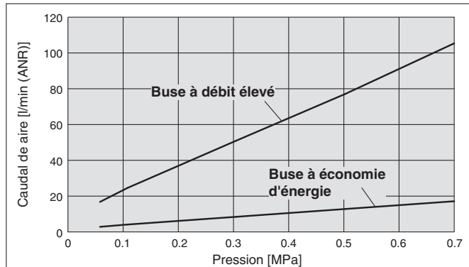
② Buse à débit élevé IZN10E-02-X367
