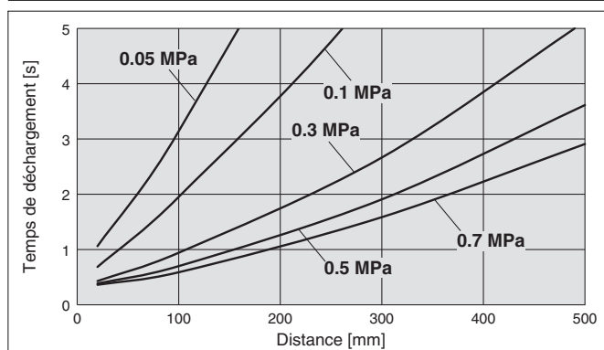
① Buse à économie d'énergie IZN10E-01-X367
