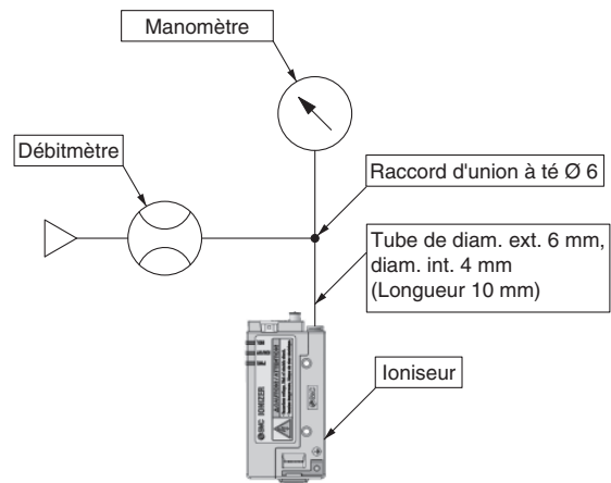
Fig. 1 : Circuit de mesure des caractéristiques du débit
