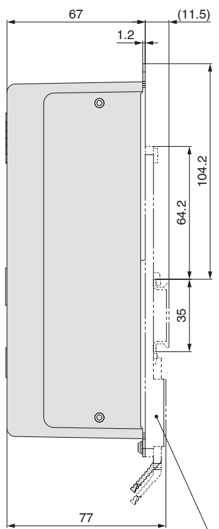
Adaptateur de montage sur rail DIN
