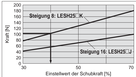
<Diagramm Einstellwert der Schubkraft–Kraft>
