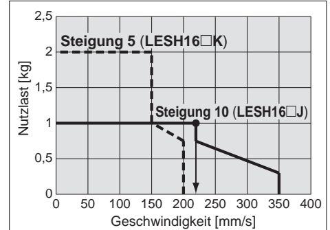
<Geschwindigkeit-Nutzlast-Diagramm>
