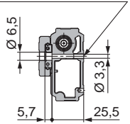
G x M4 x 0,7 Gewindetiefe 8
