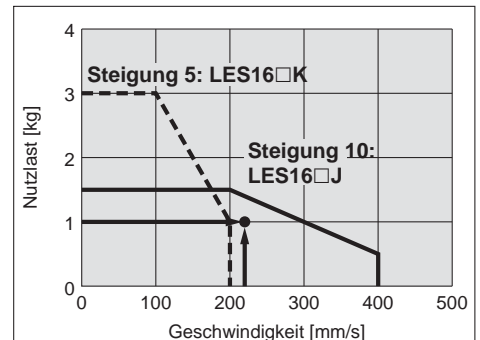
<Geschwindigkeit-Nutzlast-Diagramm>
