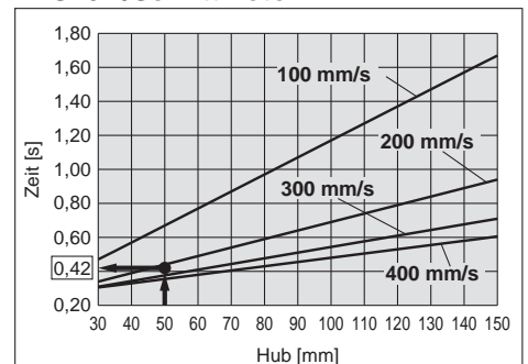
<Zykluszeit>
