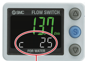
Affichage de la température
