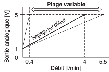
Pour modèle de 4 l/min (affichage intégré)
